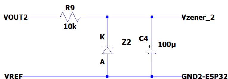
Figura 34: Circuito com filtro
