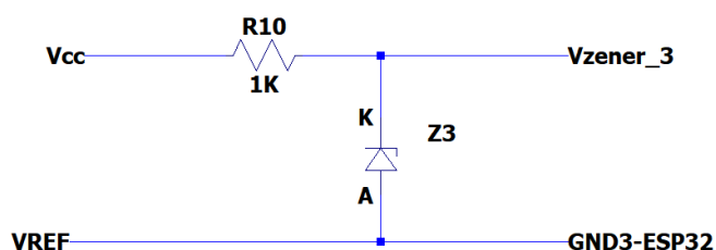
Figura 29: Circuito de segurança entrada máxima
