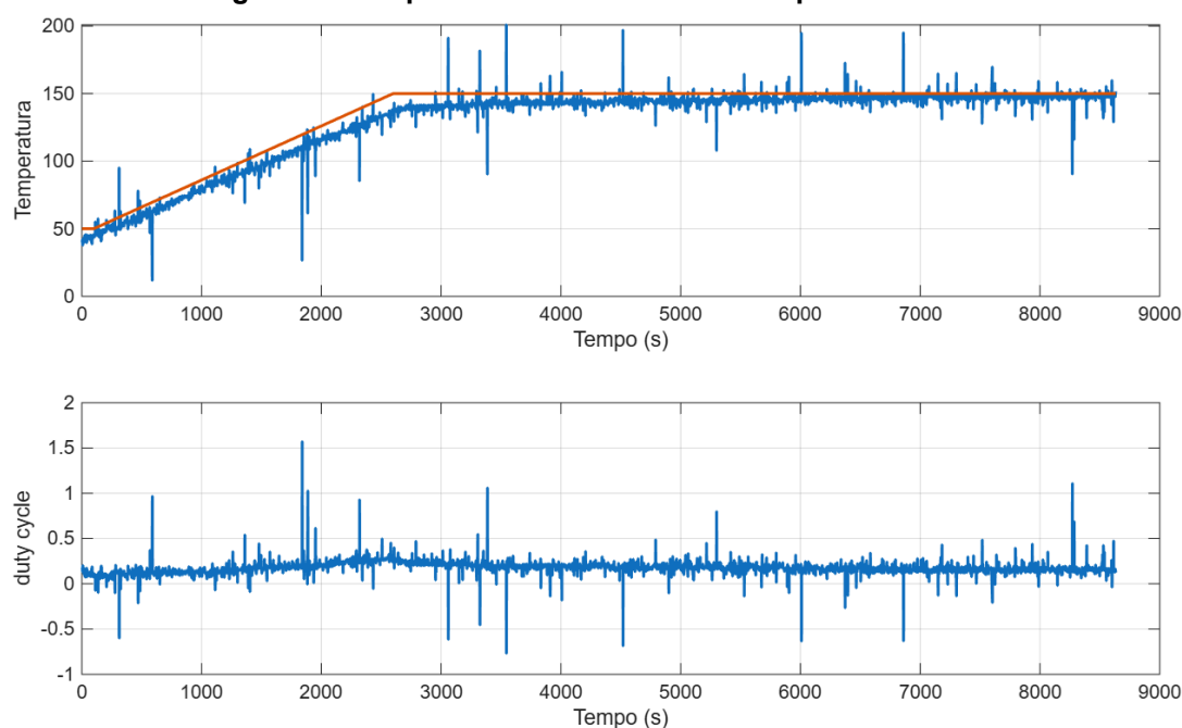
Figura 51: Resposta do sistema a uma rampa de 2°C/min
