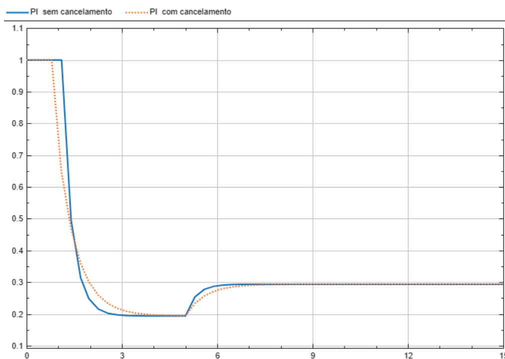
Figura 49: Esforço de controle dos controladores PI
