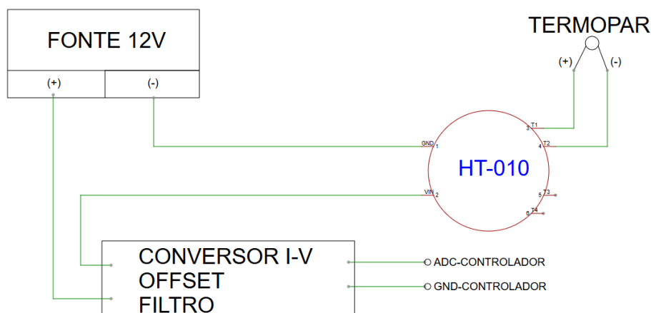
Figura 15: Cadeia de medição de temperatura
