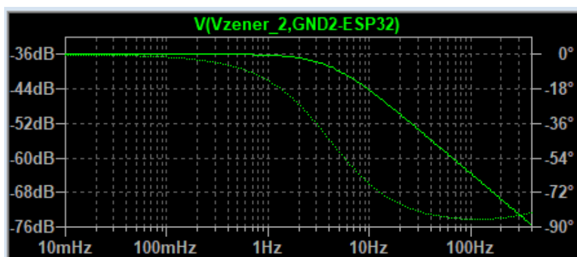
Figura 35: Simulação da resposta em frequência do filtro
