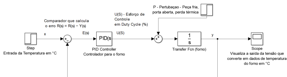
Figura 13: Sistema de controle do forno em malha fechada
