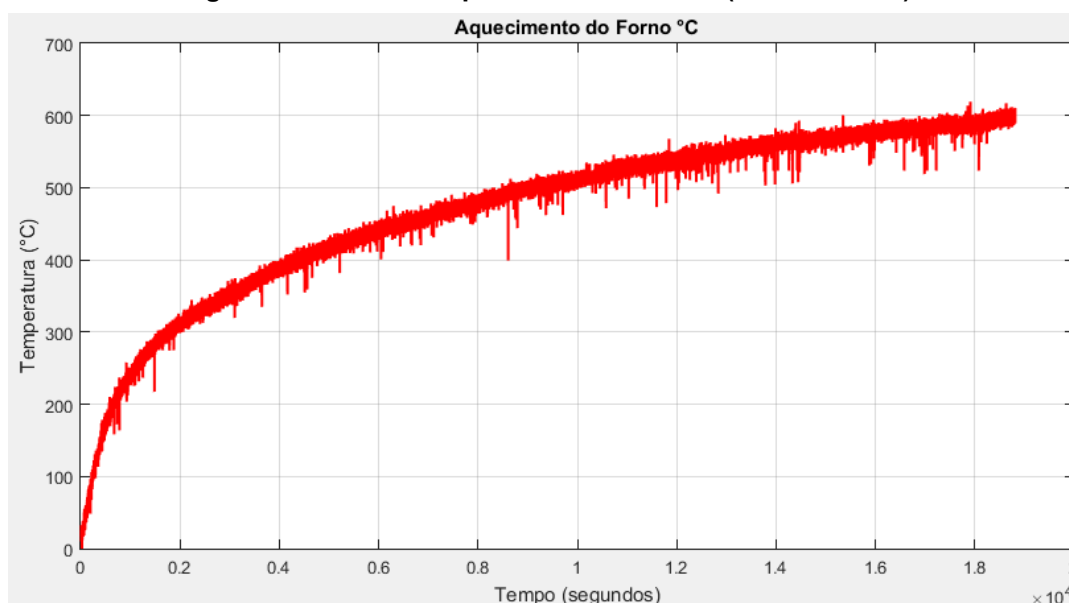
Figura 44: Curva de aquecimento do forno (dados brutos)
