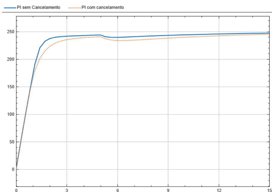
Figura 48: Entrada em degrau com perturbação em degrau
