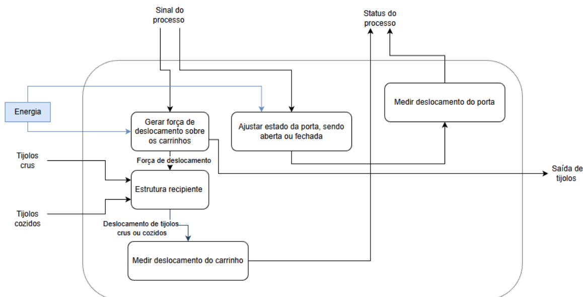
Figura 12: Transporte, entrada e saída de tijolos
