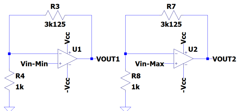
Figura 17: Entrada e a saída mínima com um amplificador ideal
