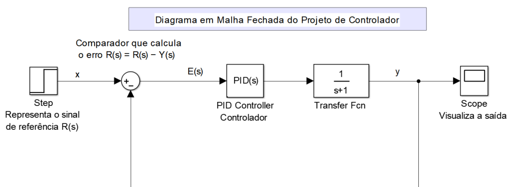
Figura 6: Diagrama de blocos
