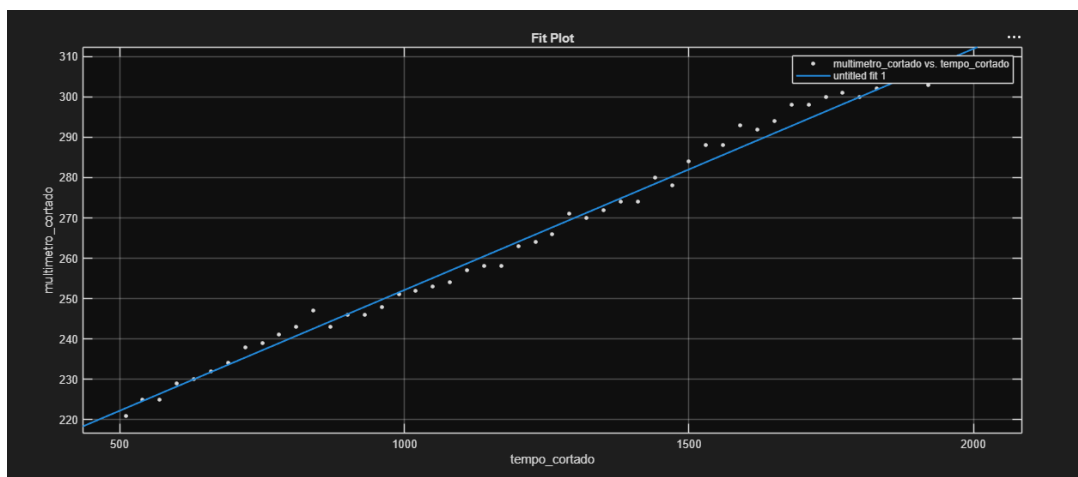
Figura 41: Interpolação dos valores do multímetro
