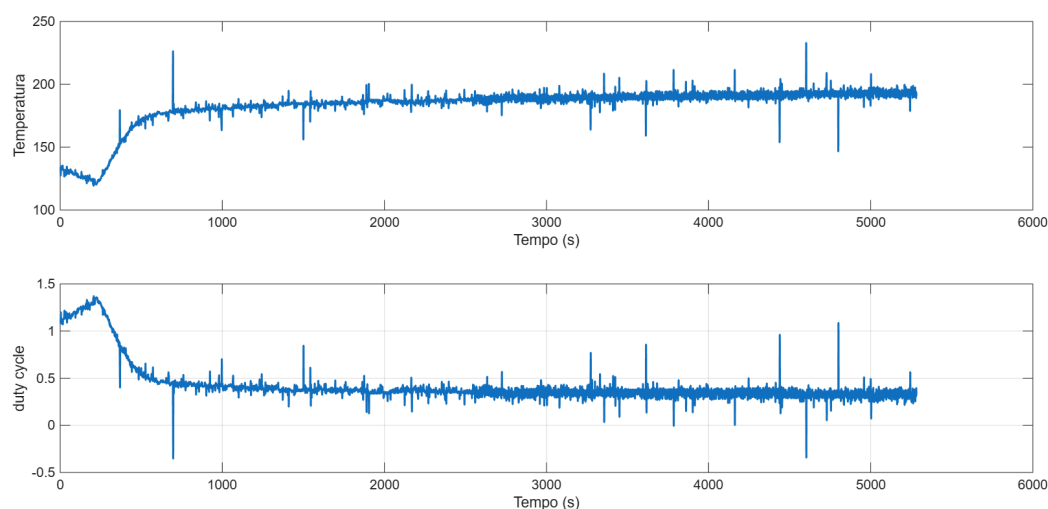
Figura 51: Resposta do sistema a uma rampa de 2°C/min
