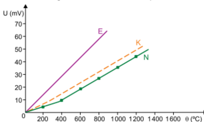
Figura 1: Sensores termopar
