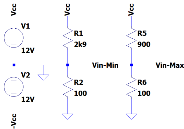
Figura 16: Divisor de Tensão
