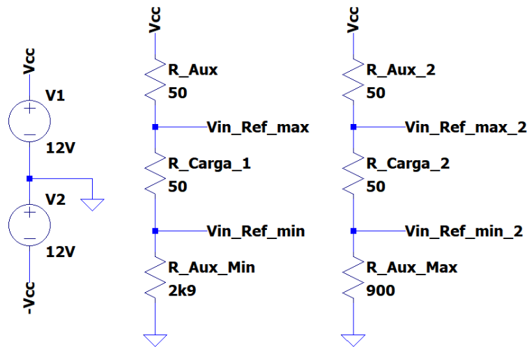
Figura 18: Divisor resistivo ajustado
