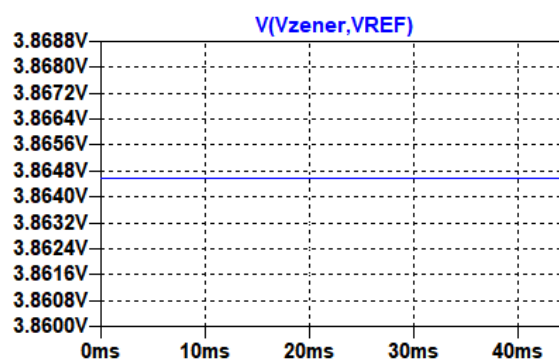
Figura 31: Simulação do circuito de segurança entrada máxima, saída
