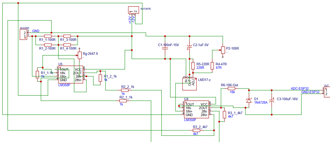
Figura 37: Esquemático da placa de condicionamento (EasyEDA)
