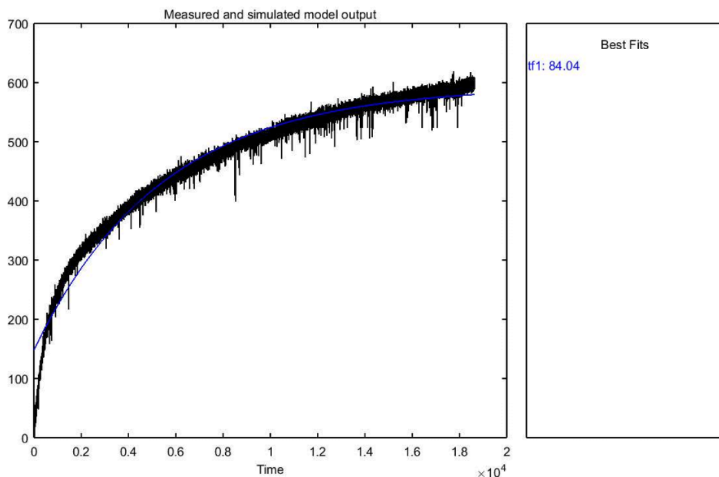
Figura 45: Identificação da planta, saída medida vs. simulada
