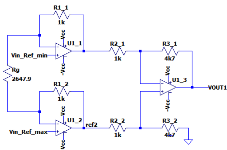
Figura 19: Amplificador de ganho, referência baixo
