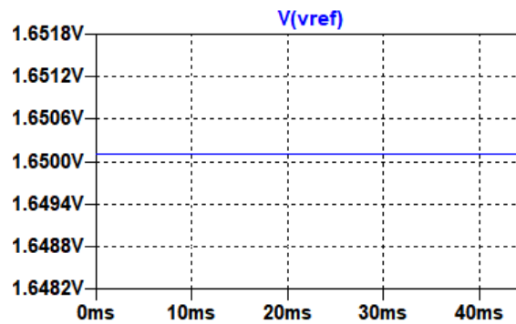
Figura 26: Simulação do circuito de offset
