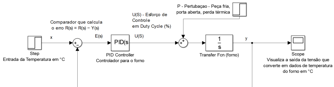
Figura 11: Controlador
