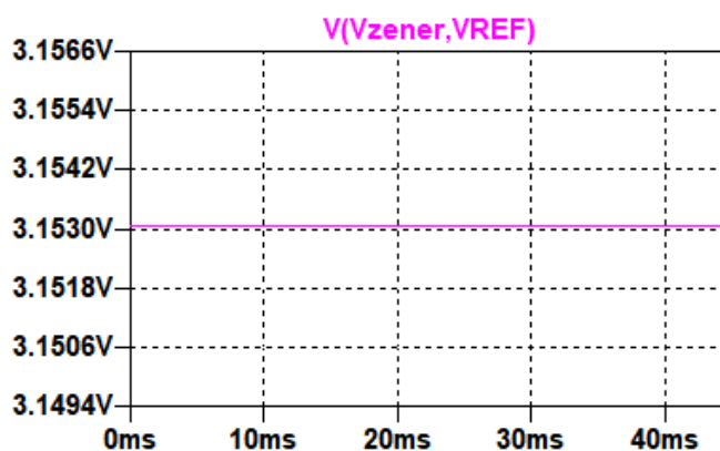
Figura 28: Simulação de circuito de segurança
